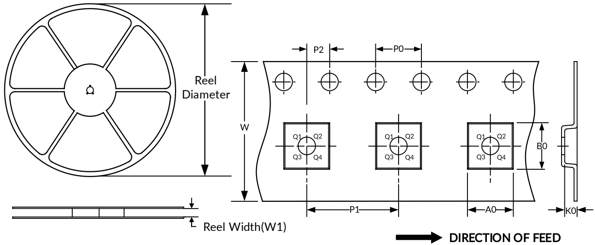
卷盘尺寸
