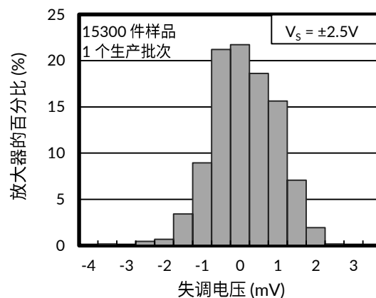
图 14. 失调电压分布
