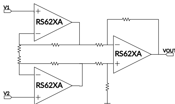
图 16. 仪表放大器
