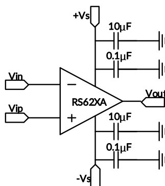
图 15. 带旁路电容器的放大器
