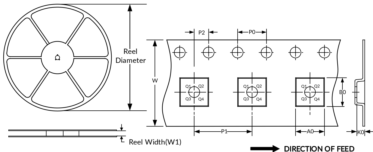
卷盘尺寸
