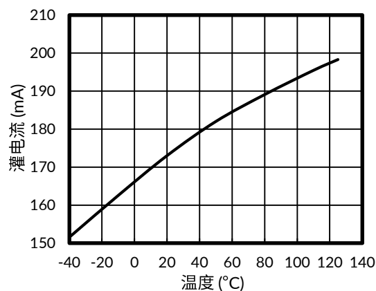
图 7. 灌电流与温度的关系
