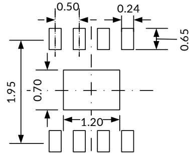
底视图
