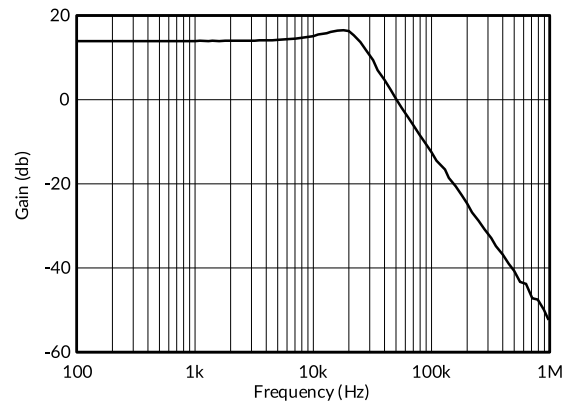
图 19. 低通滤波器
