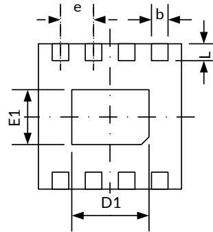
底视图
