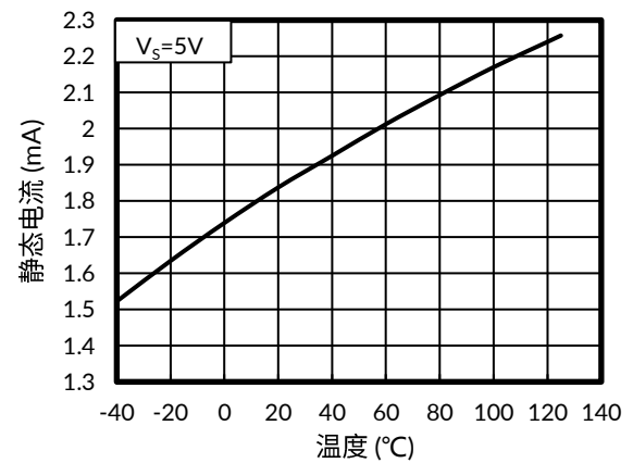
图 6. 静态电流与温度的关系
