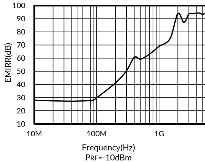
图 16. RS82X EMIRR和频率的关系
