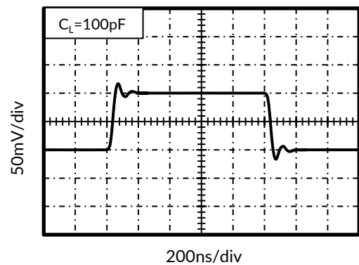
图 10. 小信号阶跃响应
