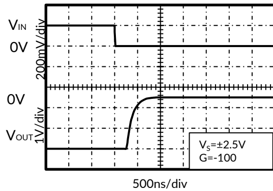
图 13. 反向过载恢复
