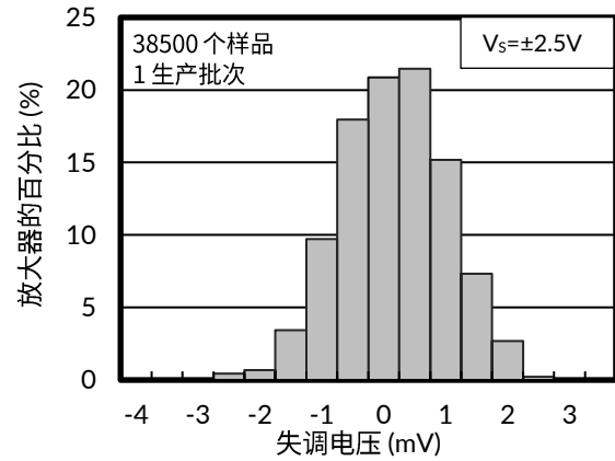
图 14. 失调电压分布
