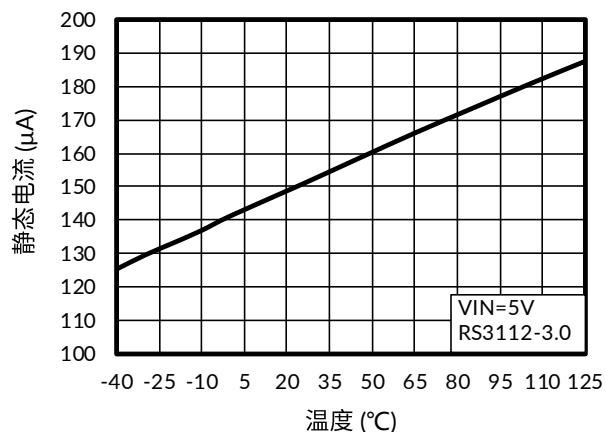
图 7. 静态电流与温度间的关系
