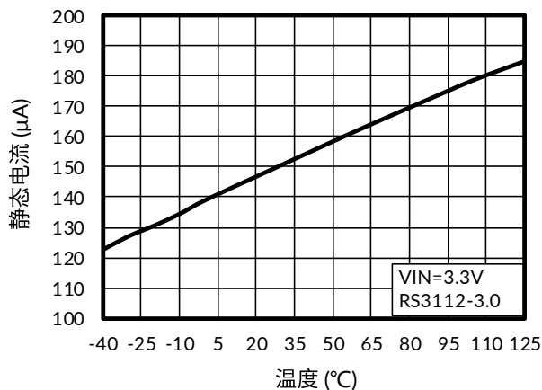
图 6. 静态电流与温度间的关系
