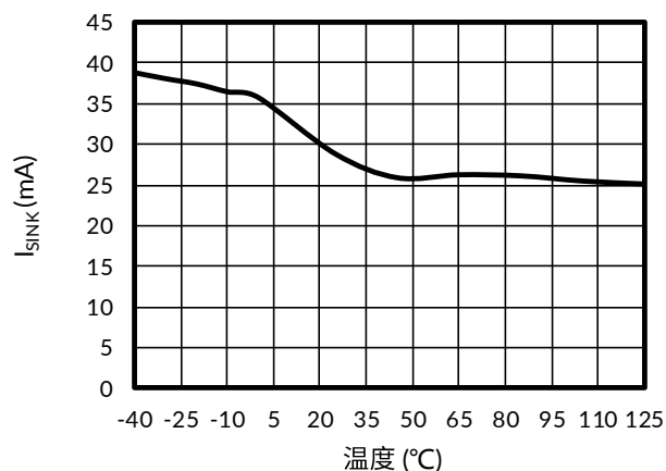
图 9. 灌电流与温度间的关系
