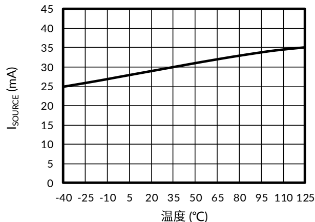
图 10. 拉电流与温度间的关系
