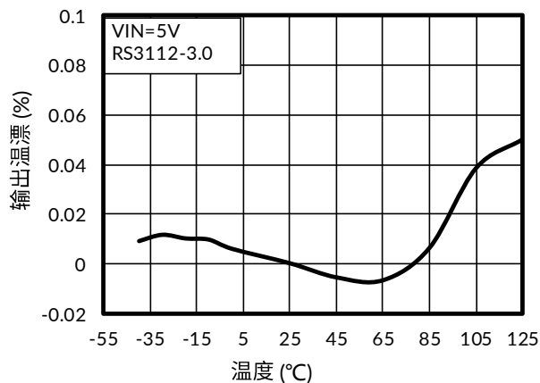
图 5. 输出电压与温度间的关系
