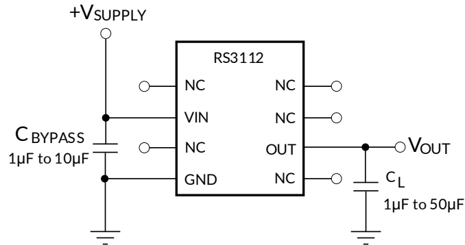
图 19. 基本连接
