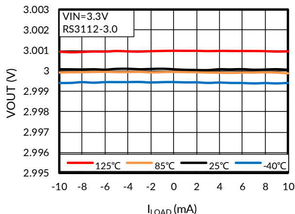
图 13. 输出电压与输出电流间的关系
