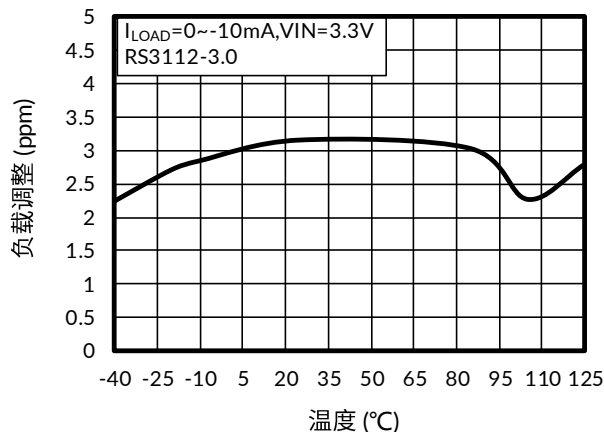
图 14. 负载调整与温度间的关系
