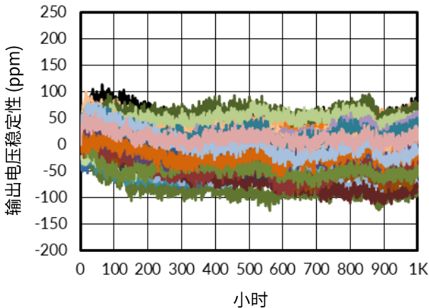
图 18. 长期稳定性 (0-1000 小时)
