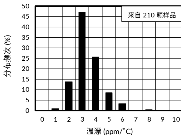
图 2. 温漂 ( -40^{\circ}\text{C} \sim 105^{\circ}\text{C} )
