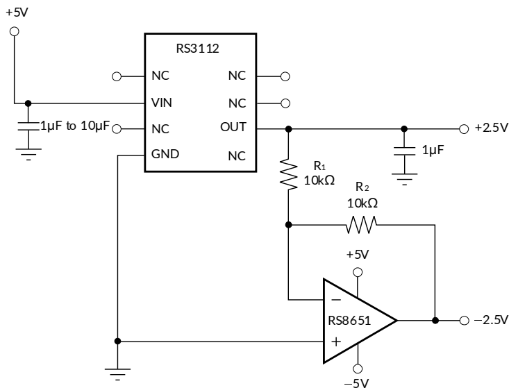
图 20. RS3112 与 RS8651 可产生正负基准电压
