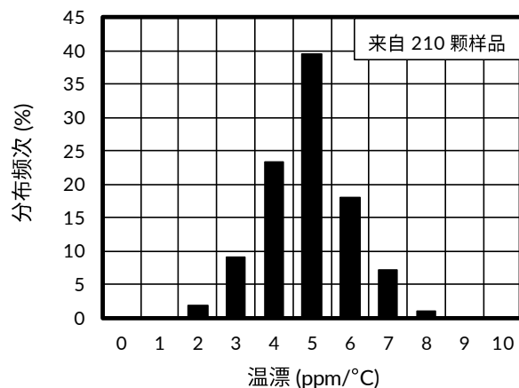
图 3. 温漂 ( -40^{\circ}\text{C} \sim 125^{\circ}\text{C} )
