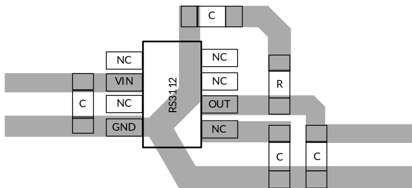
图 21. 布局示例
