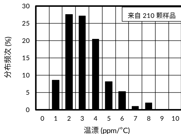
图 1. 温漂 ( 0^{\circ}\text{C} \sim 70^{\circ}\text{C} )
