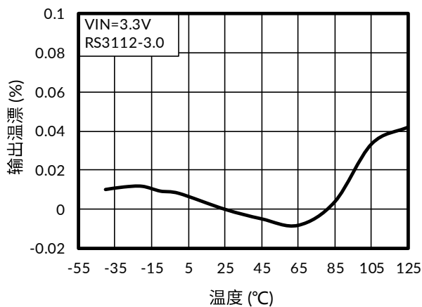
图 4. 输出电压与温度间的关系
