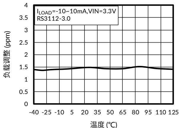
图 15. 负载调整与温度间的关系
