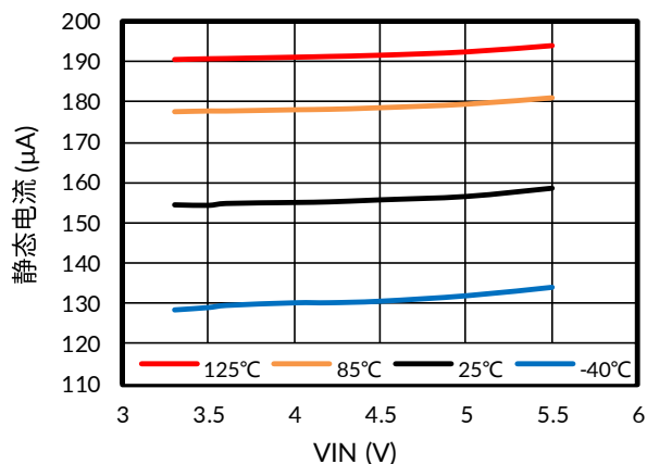
图 8. 静态电流与输入电压间的关系
