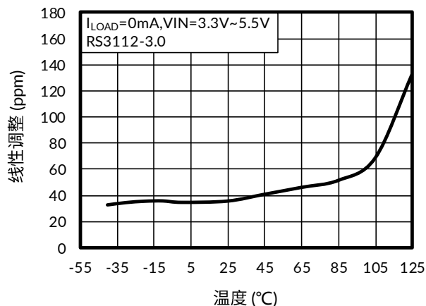
图 17. 线性调整与温度间的关系
