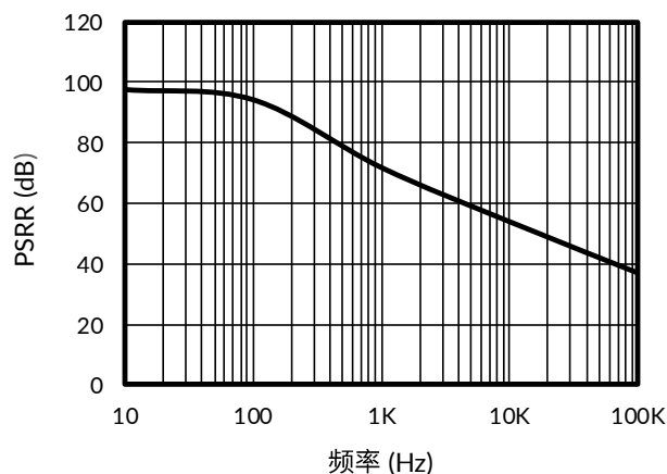
图 11. 电源抑制比与频率之间的关系
