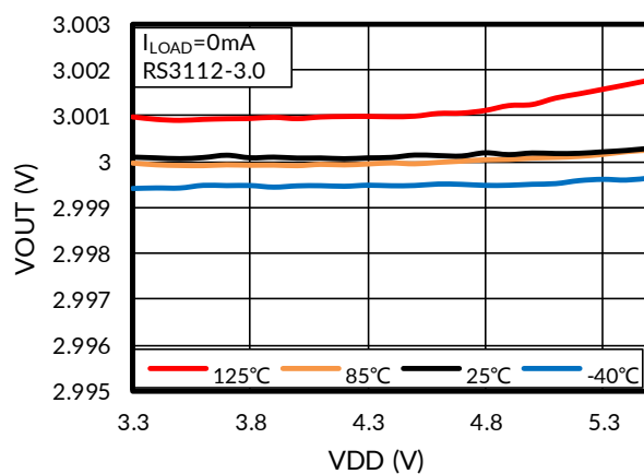
图 12. 输出电压与电源电压间的关系
