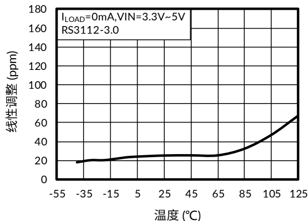
图 16. 线性调整与温度间的关系
