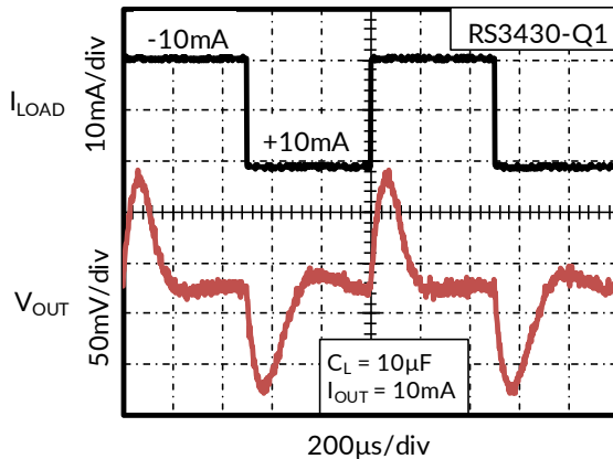
图 15. 负载调整率
