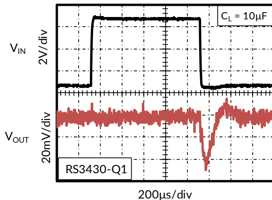
图 17. 线性调整率
