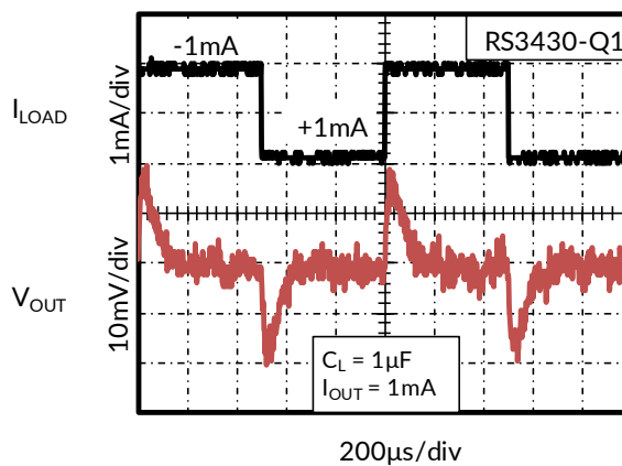
图 12. 负载调整率
