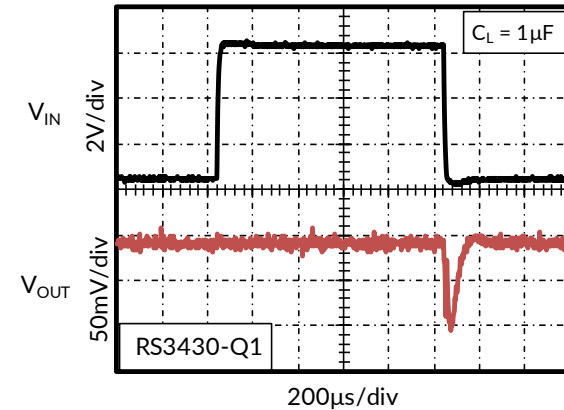
图 16. 线性调整率
