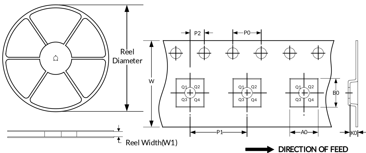
卷盘尺寸
