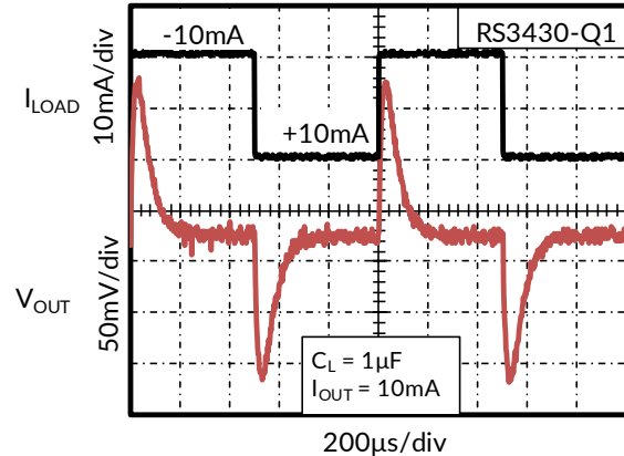
图 14. 负载调整率
