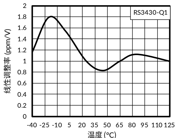
图 8. 线性调整率
