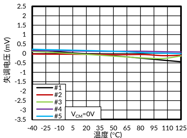
图 2. 失调电压与温度的关系
