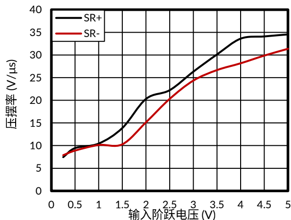
图 23. 压摆率与输入阶跃电压的关系
