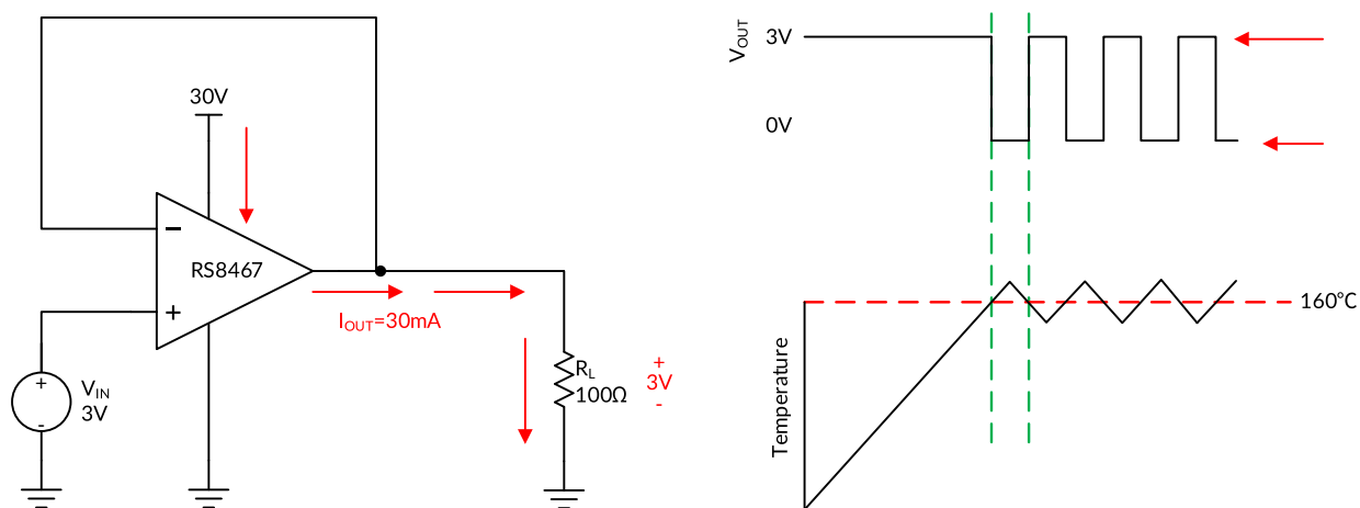
图 32. 过热保护
