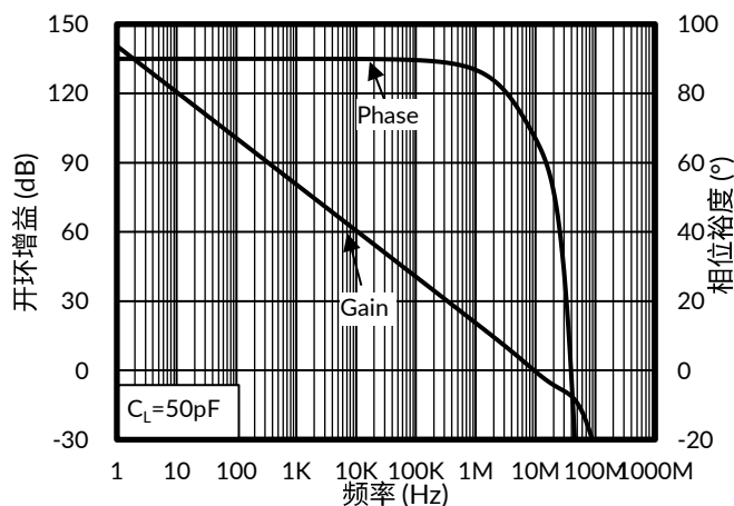
图 29. 开环增益和相位裕度与频率的关系
