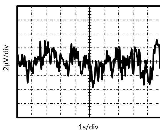
图 24. 0.1Hz~10Hz输入电压噪声
