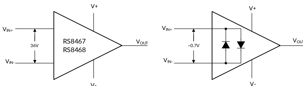
图 30. 输入保护不限制差分输入能力
