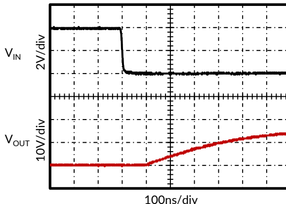
图 26. 反向过载恢复
