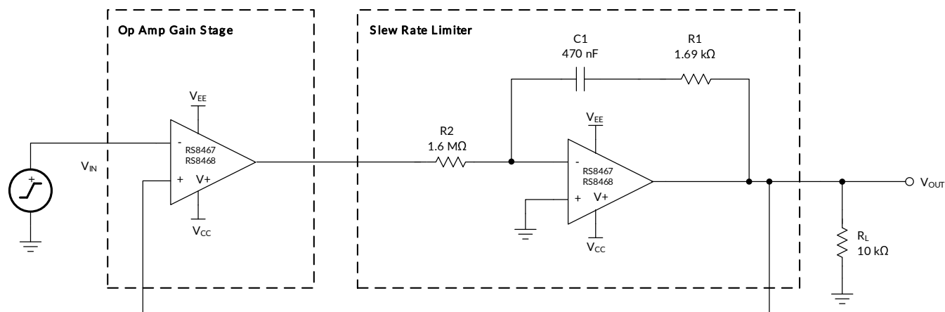
图 35. 压摆率限制器使用一个运算放大器
