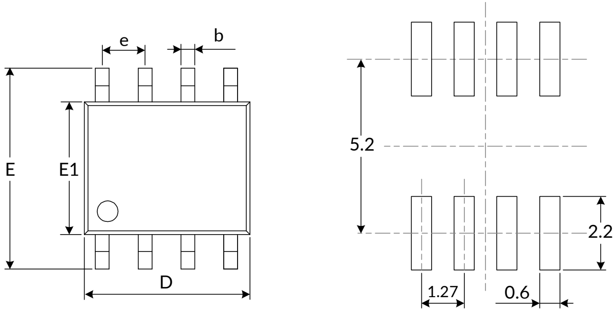
推荐焊盘尺寸 (单位: 毫米)
