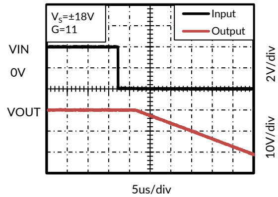
图 8. 反向过载恢复
