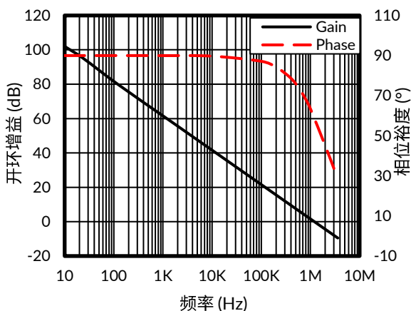
图 1. 开环增益和相位裕度与频率的关系
