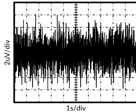
图 10. 0.1Hz~10Hz 输入电压噪声 AT V_S = 5\text{V}
