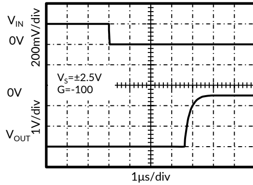
图 13. 反向过载恢复
