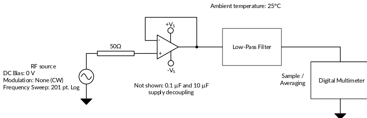
图 16. EMIRR IN+ 测试配置示意图
