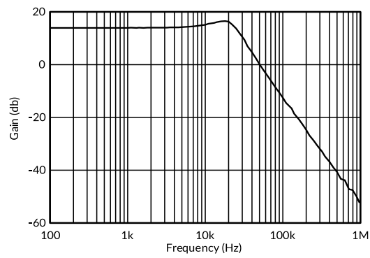
图 18. 低通滤波器
