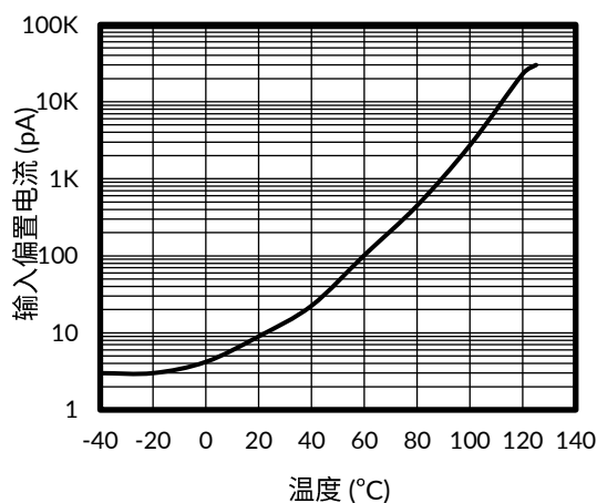
图 9. 输入偏置电流与温度的关系
