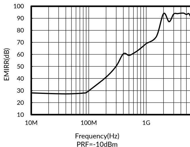
图 15. RS633XP EMIRR和频率的关系
