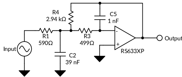
图 17. 25-kHz 低通滤波器
