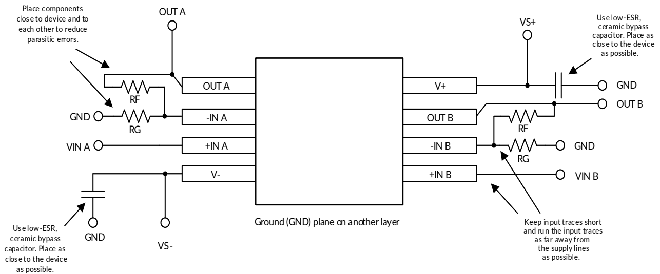
图 20. PCB 布局建议
