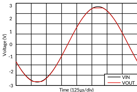
图 14. 在输入过驱动状态下无相位翻转的输出波形
