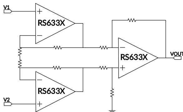
图 16. 仪表放大器
