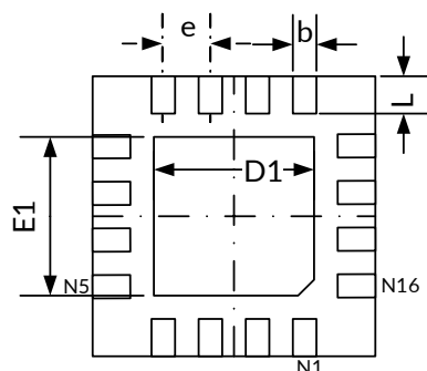
底视图
