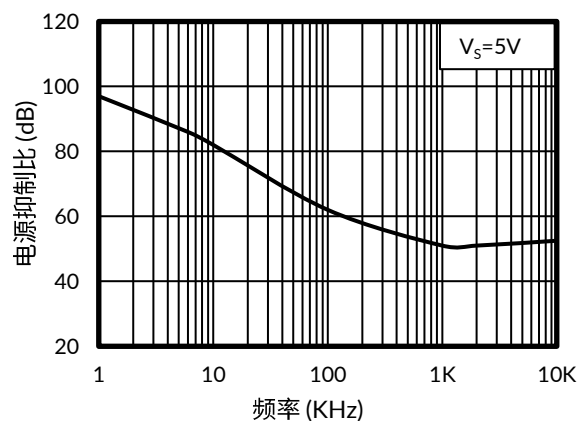
图 4. 电源抑制比与频率的关系
