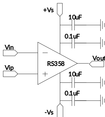
图 14. 带旁路电容器的放大器
