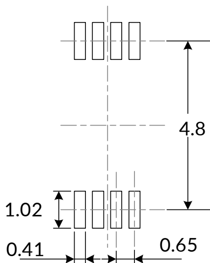
推荐焊盘尺寸 (单位: 毫米)
