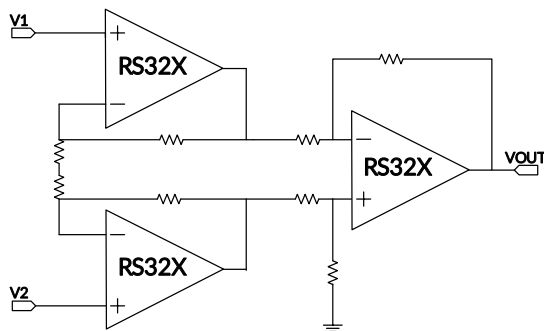
图 15. 仪表放大器
