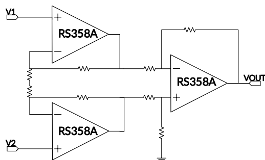
图 15. 仪表放大器
