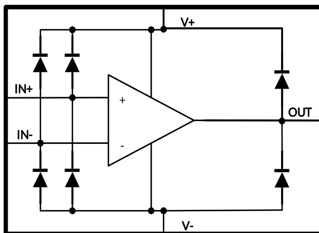
图 16. 功能框图
