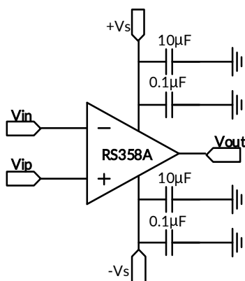
图 14. 带旁路电容器的放大器
