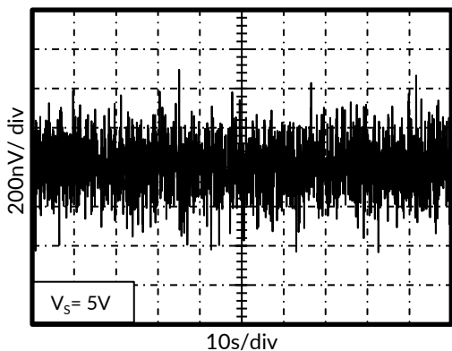
图 15. 0.01Hz ~ 10Hz 输入电压噪声
