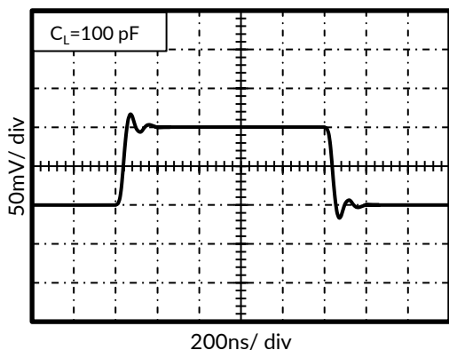
图 11. 小信号阶跃响应
