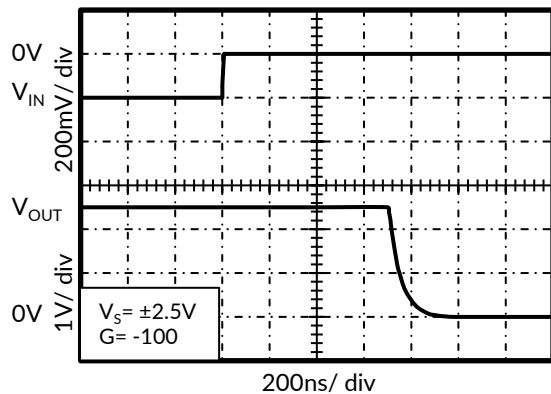
图 13. 正向过载恢复
