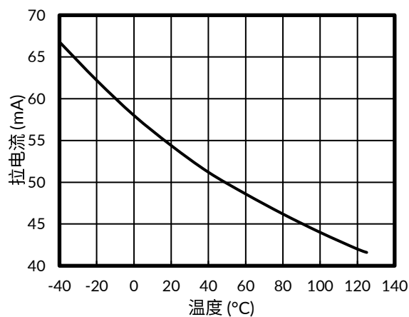
图 9. 拉电流与温度的关系
