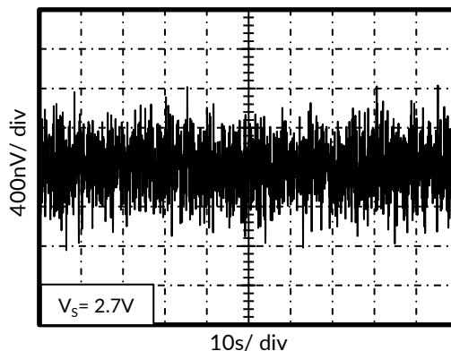
图 16. 0.01Hz ~ 10Hz 输入电压噪声
