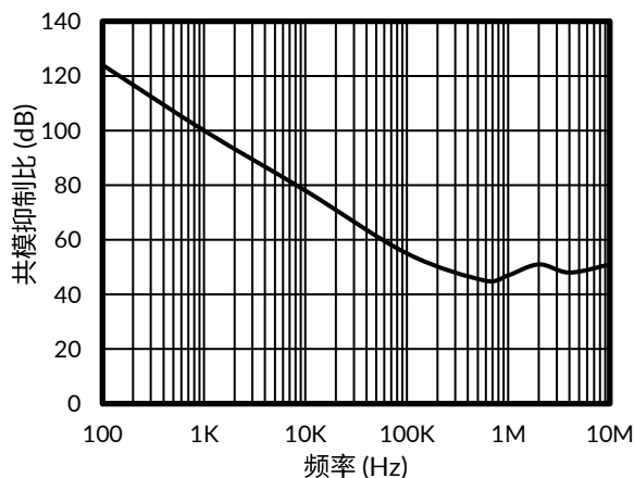
图 6. 共模抑制比与频率的关系
