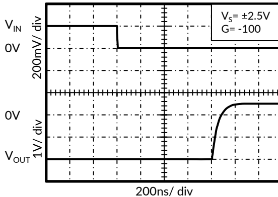
图 14. 反向过载恢复
