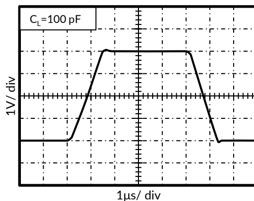
图 12. 大信号阶跃响应
