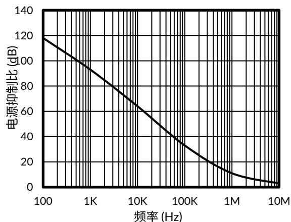
图 5. 电源抑制比与频率的关系
