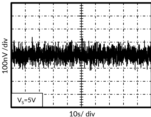
图 17. 0.01Hz ~ 1Hz 输入电压噪声
