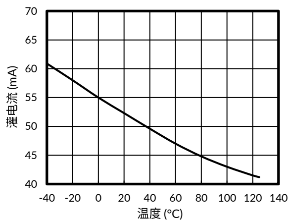
图 10. 灌电流与温度的关系
