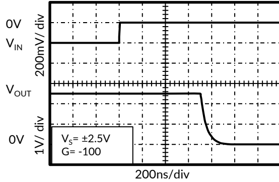
图 13. 正向过载恢复
