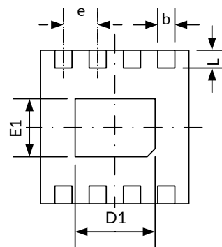
底视图
