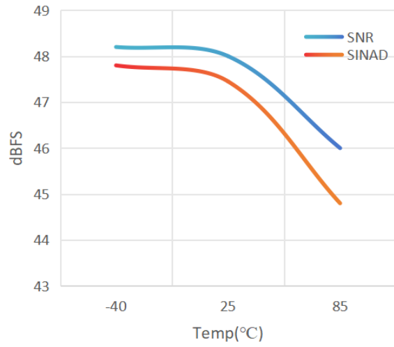
图 10. SNR/SINAD 与温度关系
