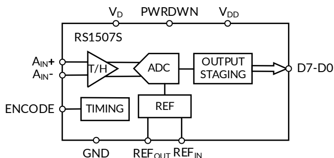
图 1. RS1507S 框图
