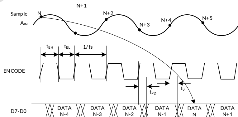
图 2. 时序图
