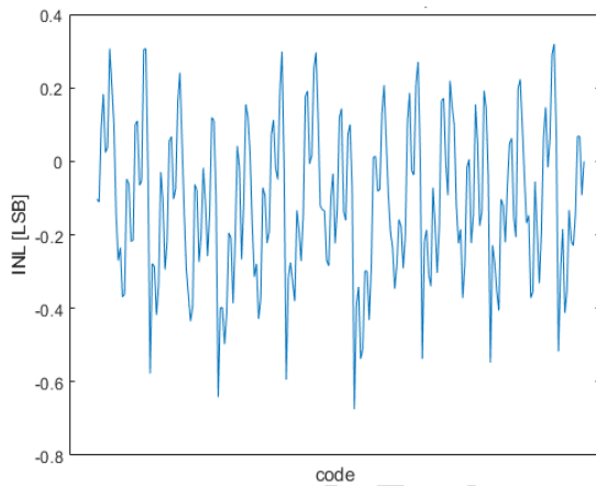
图 11. 积分非线性
