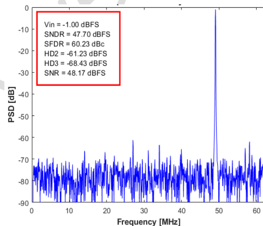
图 6. 输入信号 76MHz 单音频谱
