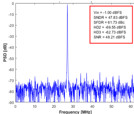
图 4. 输入信号 26MHz 单音频谱
