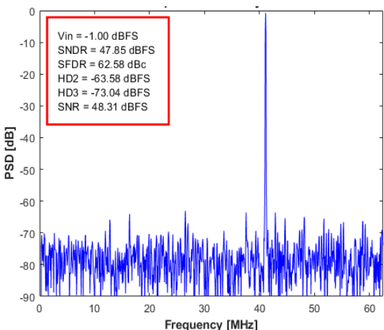
图 5. 输入信号 41MHz 单音频谱
