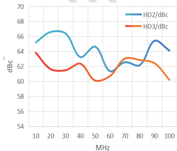
图 7. 二三次谐波与输入信号关系
