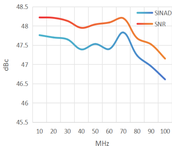
图 8. SNR/SINAD 与输入信号关系
