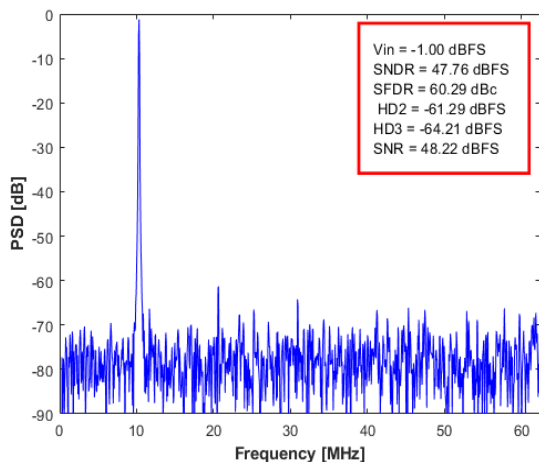
图 3. 输入信号 10.3MHz 单音频谱
