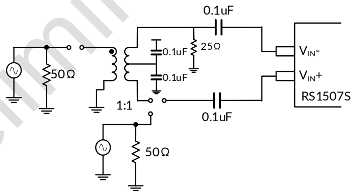
图 13. 模拟信号输入应用原理图
