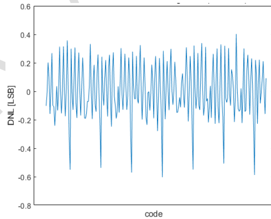
图 12. 微分非线性
