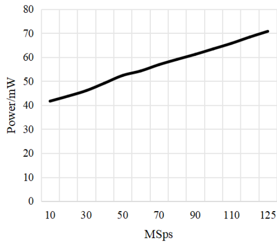
图 9. DC 输入功耗与采样率的关系
