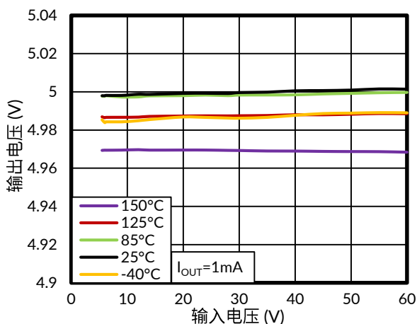
图 8. 线性调整率
