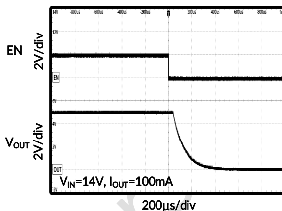
图 26. 关断时序
