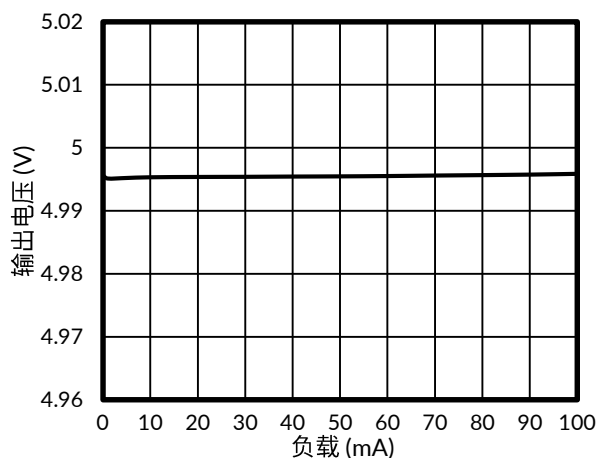
图 7. 负载调整率
