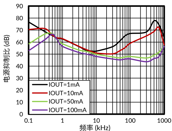
图 11. 电源抑制比与频率的关系
