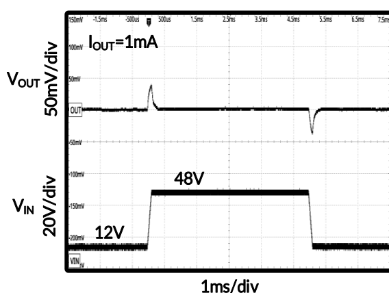
图 30. 线性瞬态响应
