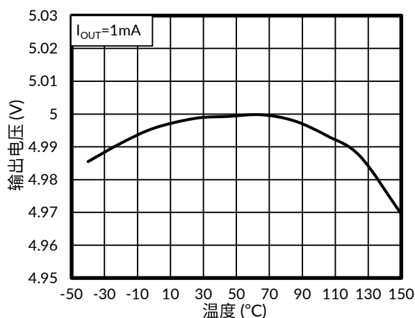
图 9. 输出电压与温度的关系
