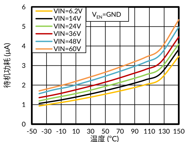
图 4. 待机功耗与温度的关系
