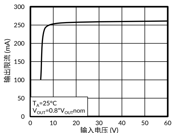
图 17. 输出限流与输入电压的关系
