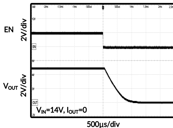
图 24. 关断时序
