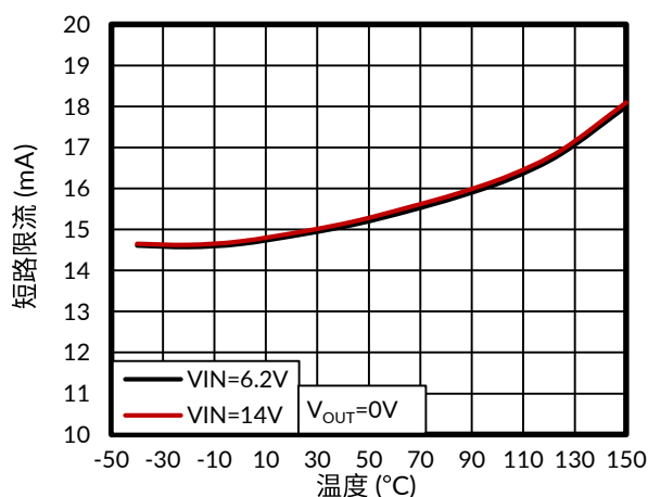
图 16. 短路限流与温度的关系
