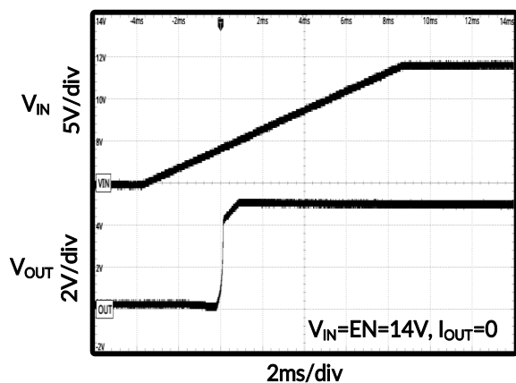
图 19. 上电时序
