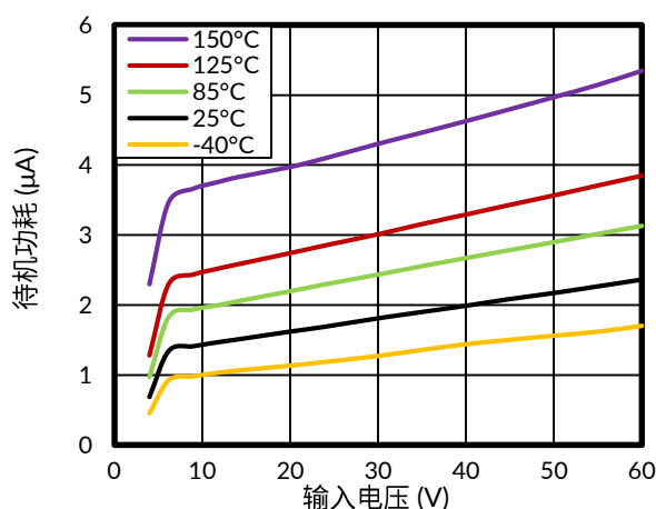
图 3. 待机功耗与输入电压的关系
