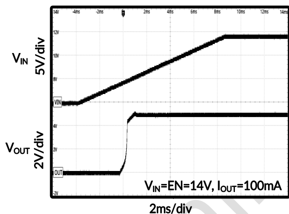
图 21. 上电时序
