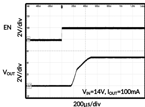
图 25. 开启时序
