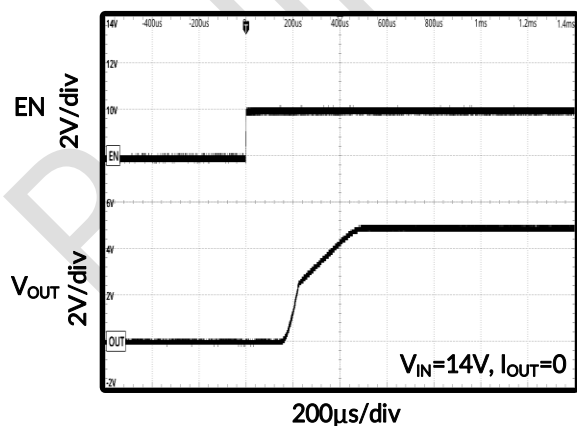
图 23. 开启时序
