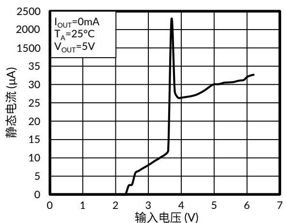
图 5. 静态电流与输入电压的关系
