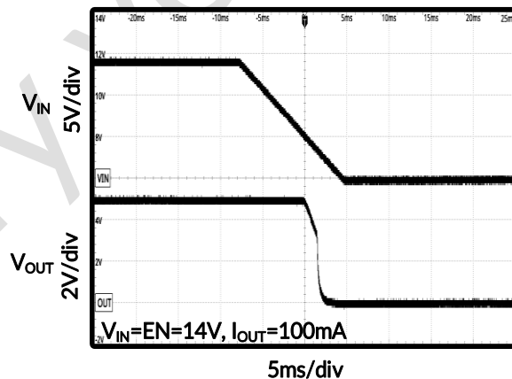
图 22. 下电时序
