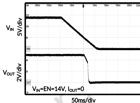
图 20. 下电时序
