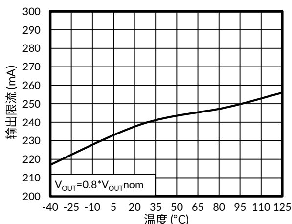
图 18. 输出限流与温度的关系
