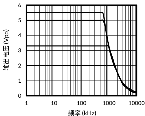
图 17. 闭环输出电压摆幅
