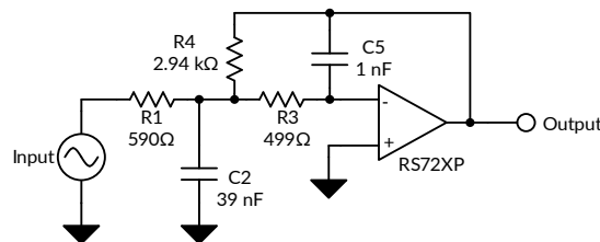
图 25. 25-kHz 低通滤波器
