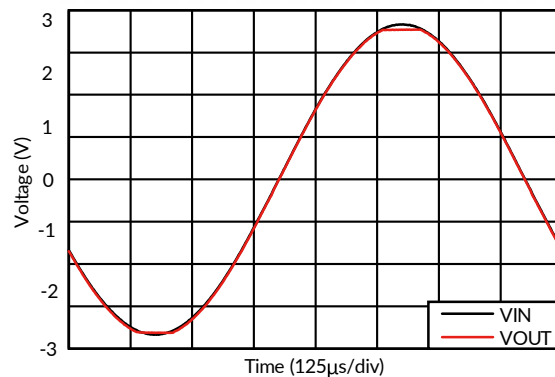
图 22. 在输入过驱动状态下无相位翻转的输出波形
