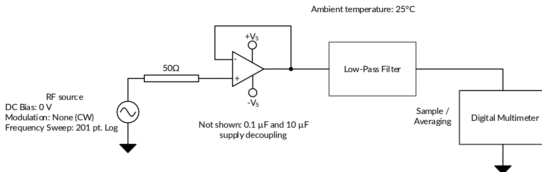
图 24. EMIRR IN+ 测试配置示意图
