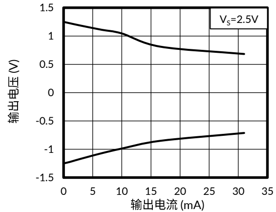
图 20. 输出电压与输出电流的关系
