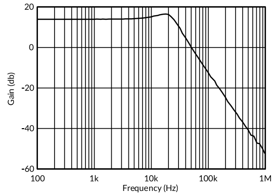
图 26. 低通滤波器
