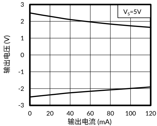
图 19. 输出电压与输出电流的关系
