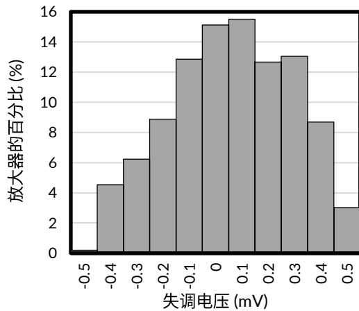
图 21. 失调电压分布
