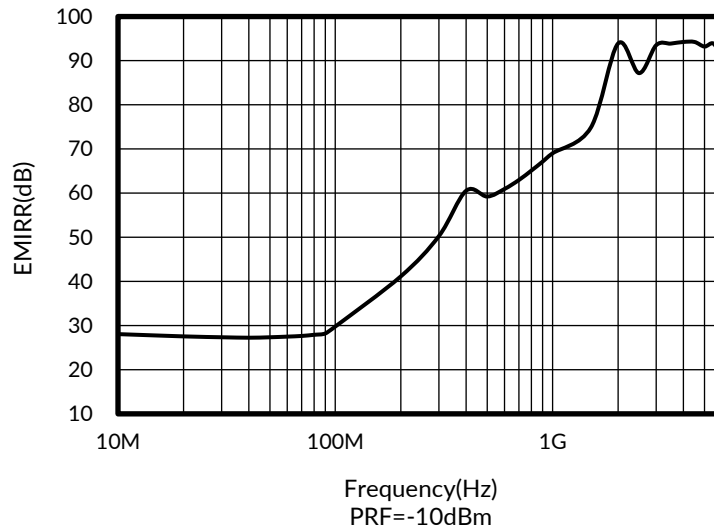
图 23. RS72XP EMIRR和频率的关系
