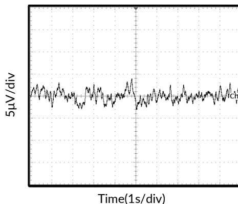
图 12. 0.1Hz~10Hz 输入电压噪声
