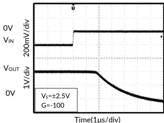
图 13. 正向过载恢复
