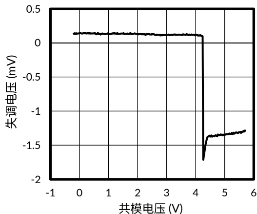
图 11. 失调电压与共模电压的关系
