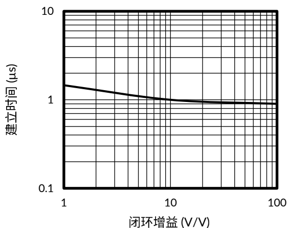
图 18. 建立时间与闭环增益的关系
