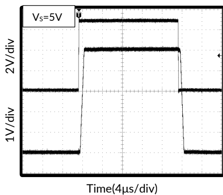
图 15. 大信号阶跃响应
