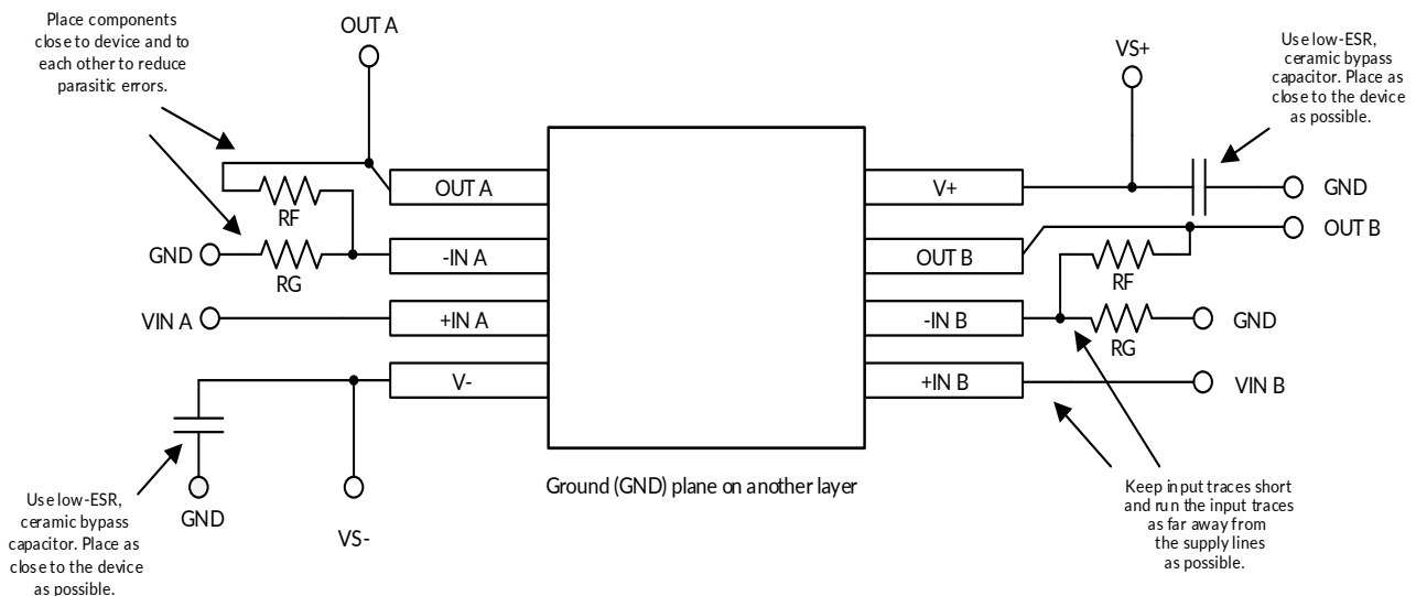
图 28. PCB 布局建议
