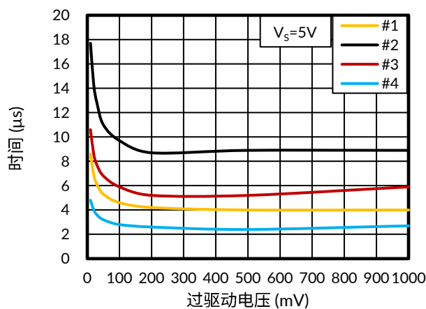
图 3. 响应时间与输入过驱动电压的关系（负向跳变）
