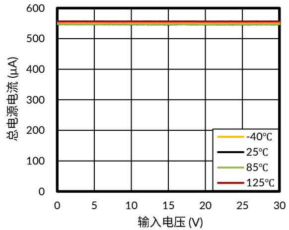
图 10. 总电源电流与输入电压的关系, 32V
