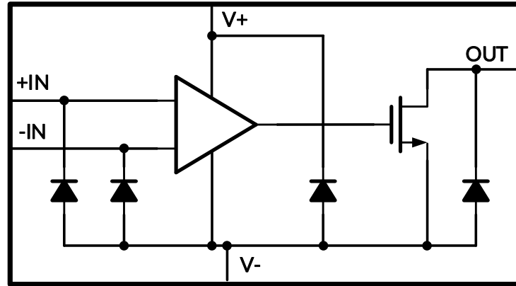
图 23. 功能框图
