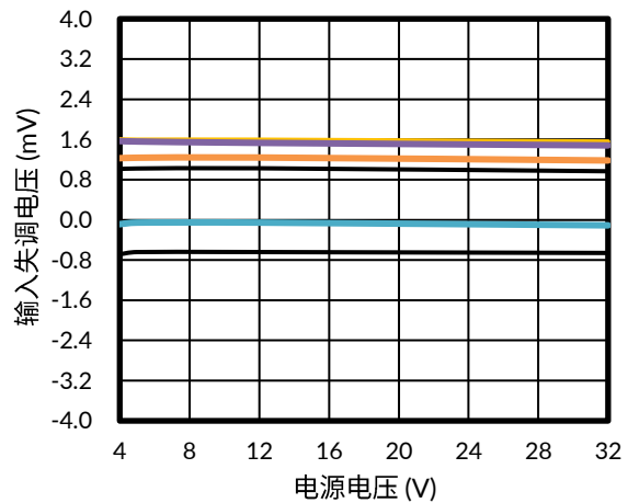
图 16. 输入失调电压与电源电压的关系, 85°C
