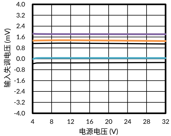
图 14. 输入失调电压与电源电压的关系, -40°C
