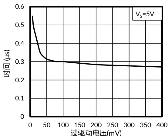
图 3. 响应时间与输入过驱动电压的关系 (负向跳变)
