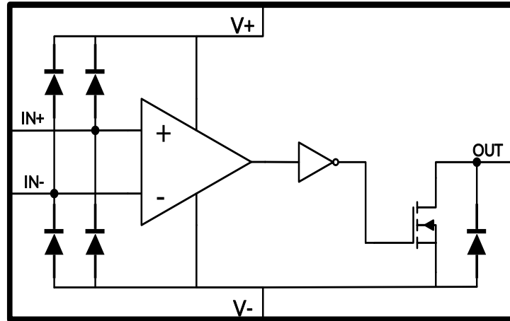
图 7. 功能框图
