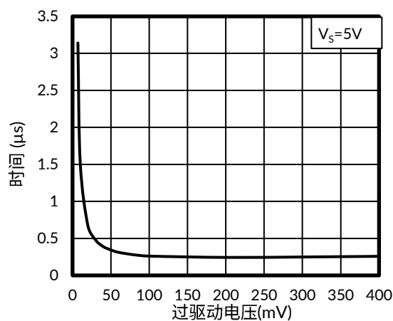
图 4. 响应时间与输入过驱动电压的关系 (正向跳变)
