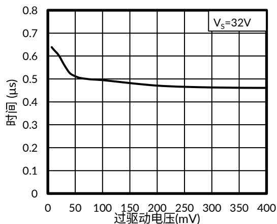
图 5. 响应时间与输入过驱动电压的关系 (负向跳变)
