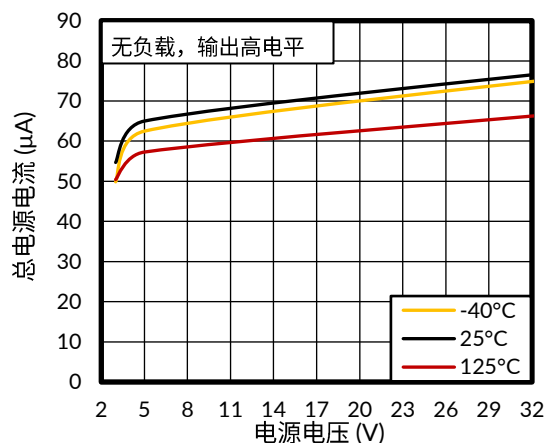
图 1. 总电源电流与电源电压的关系
