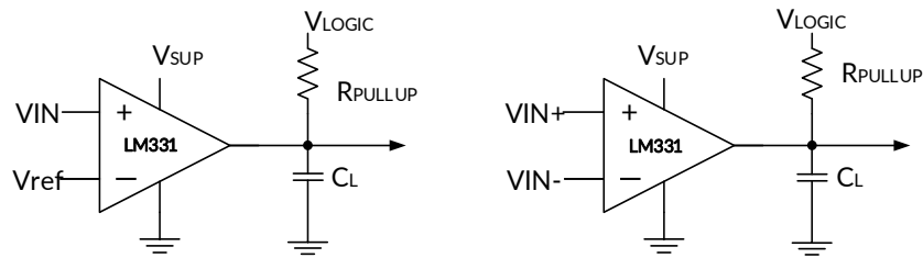
图 8. 单端和差分输入配置电路
