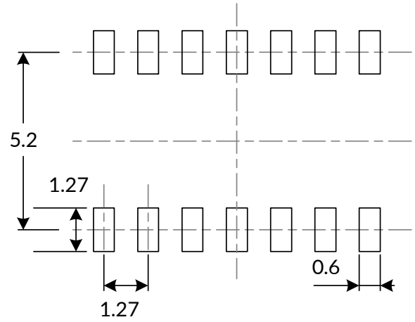
推荐焊盘尺寸 (单位: 毫米)
