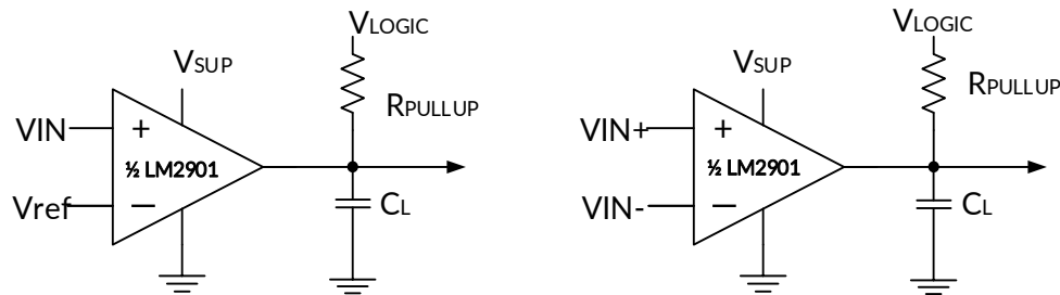
图 8. 单端和差分输入配置电路
