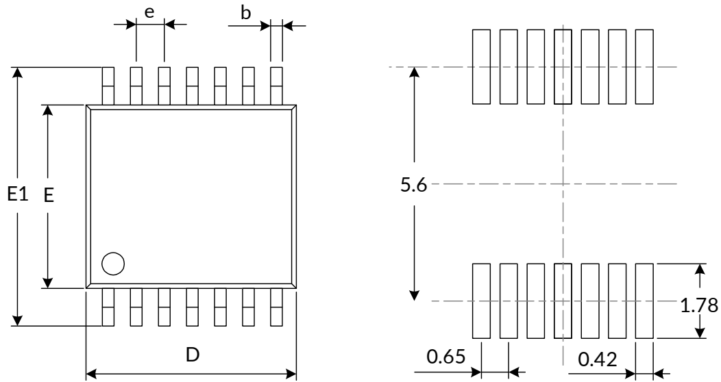
推荐焊盘尺寸 (单位: 毫米)
