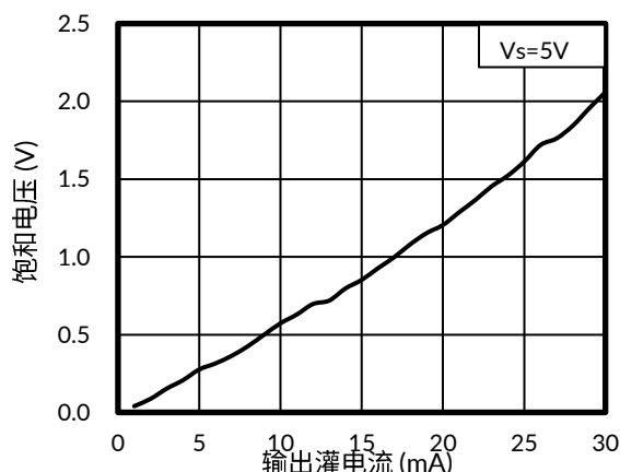
图 5. 饱和电压与输出灌电流的关系
