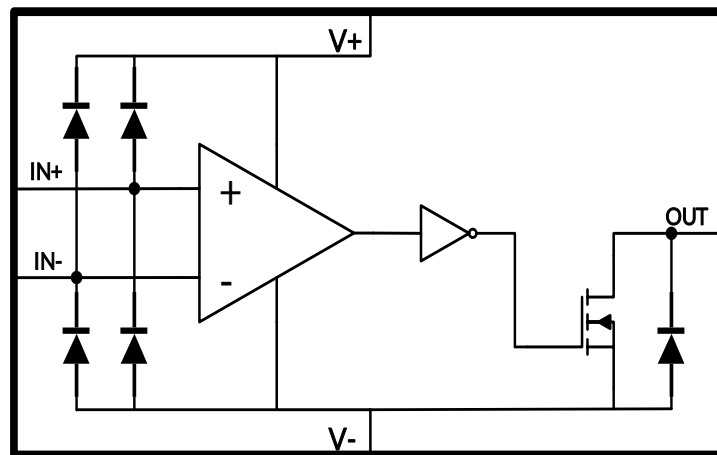
图 7. 功能框图
