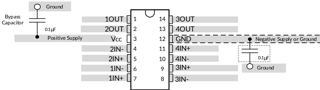
图 9. LM2901 PCB 布局示例
