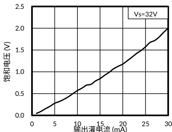
图 6. 饱和电压与输出灌电流的关系
