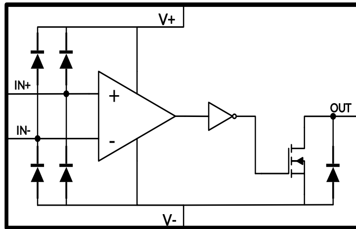
图 7. 功能框图
