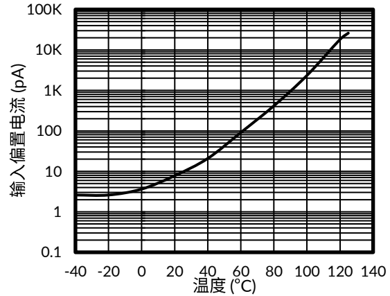
图 2. 输入偏置电流与温度的关系
