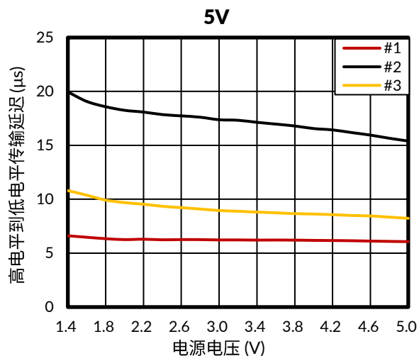
图 33. 高电平到低电平传输延迟与电源电压的关系
