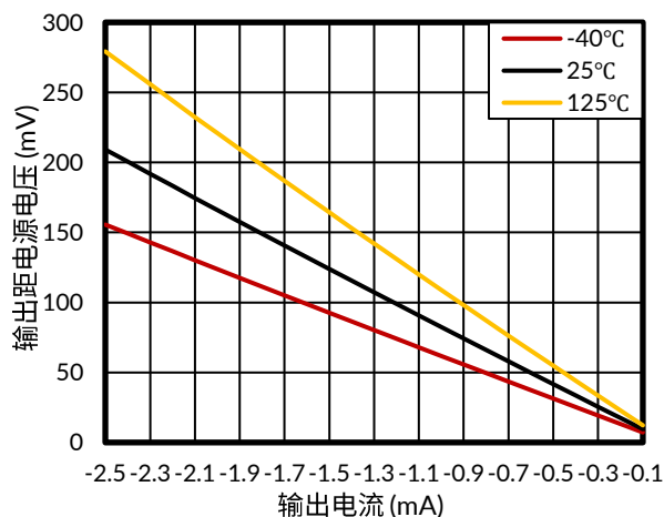
图 15. 输出电压与输出电流的关系, 3.3V
