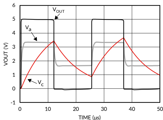
图 36. 方波振荡器输出波形图
