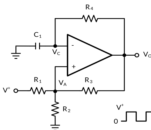
图 34. 方波发生器原理图
