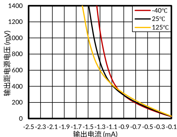
图 13. 输出电压与输出电流的关系, 1.4V
