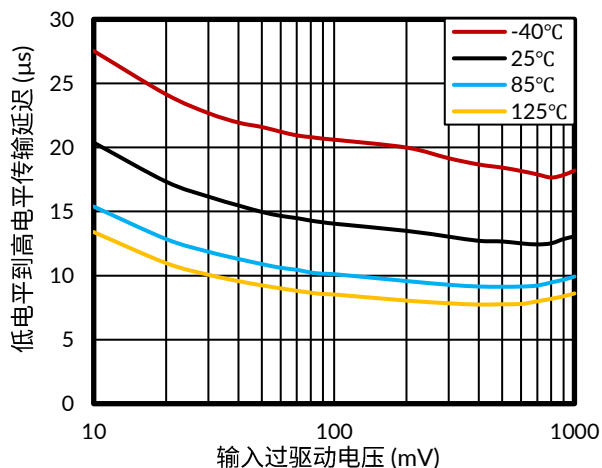
图 22. 低电平到高电平传输延迟, 5V
