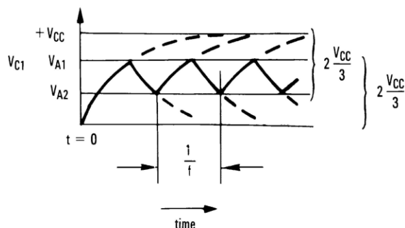
图 35. 方波振荡器
