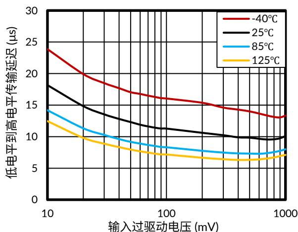
图 21. 低电平到高电平传输延迟, 3.3V
