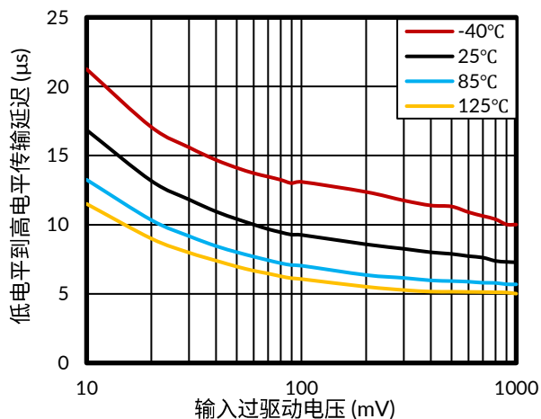
图 20. 低电平到高电平传输延迟, 1.4V
