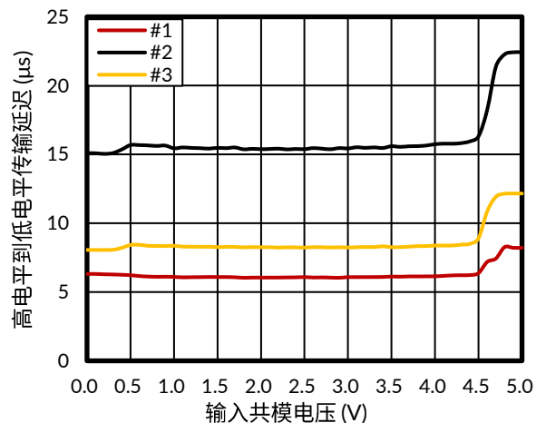
图 31. 高电平到低电平传输延迟与共模电压的关系,
