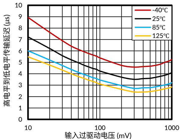
图 24. 高电平到低电平传输延迟, 3.3V
