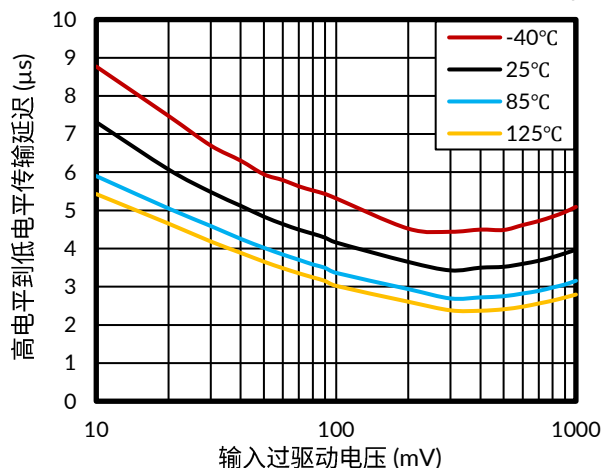
图 25. 高电平到低电平传输延迟, 5V
