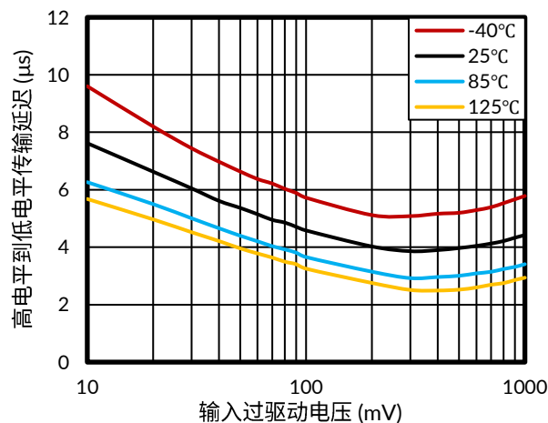
图 23. 高电平到低电平传输延迟, 1.4V
