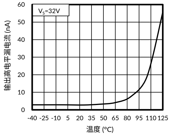
图 22. 输出高电平漏电流与温度的关系
