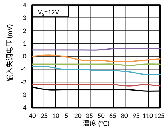
图 12. 输入失调电压与温度的关系
