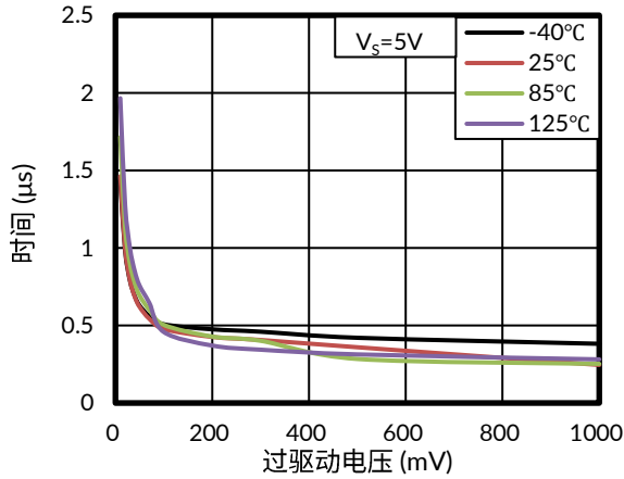
图 1. 响应时间与输入过驱动电压的关系 (负向跳变)
