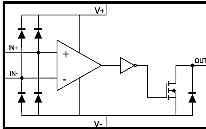
图 23. 功能框图
