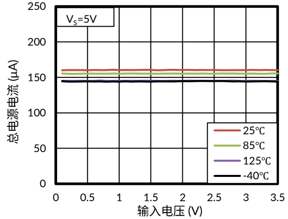
图 8. 总电源电流与输入电压的关系
