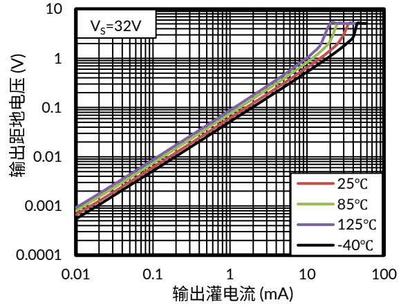
图 20. 输出低电压与输出灌电流的关系
