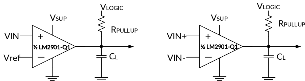
图 24. 单端和差分输入配置电路
