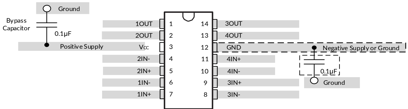
图 25. LM2901-Q1 PCB 布局示例
