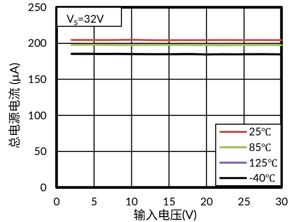
图 10. 总电源电流与输入电压的关系
