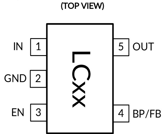
SOT23-5/SC70-5
